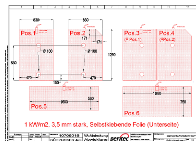
Bauelementeanordnung
