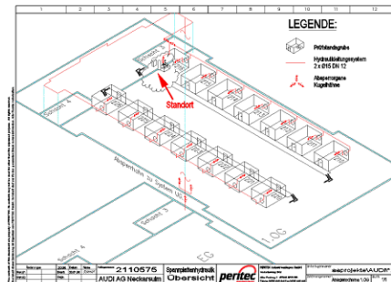
Aufstellungs- schema
