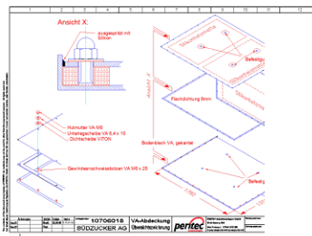
Explosionszeichnung
