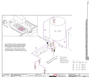
Verlegeschema
